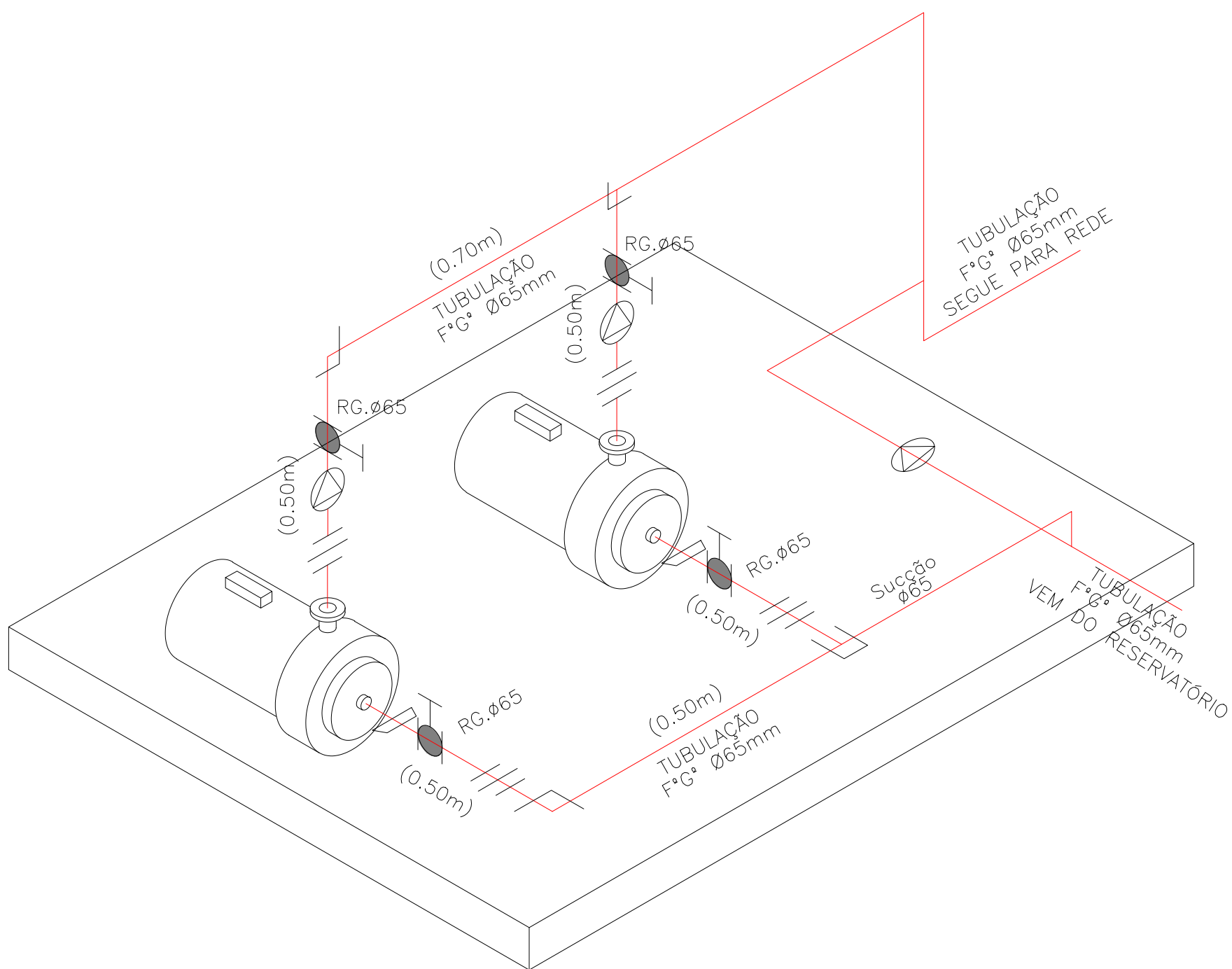
DETALHE DA BOMBA - SHP SEM ESCALA
