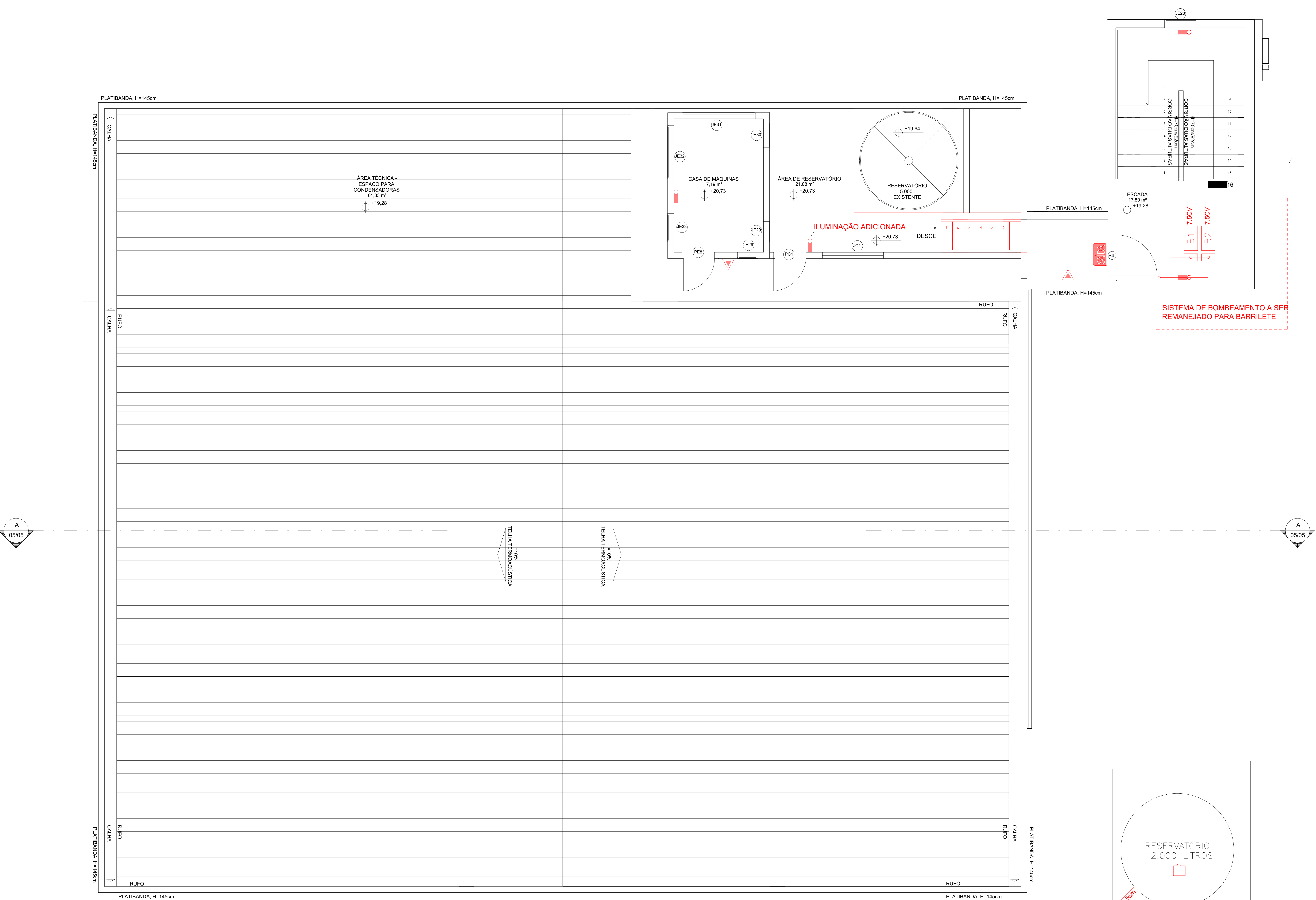
3 PLANTA RESERVATÓRIO - ALTERAÇÃO 1 : 50
